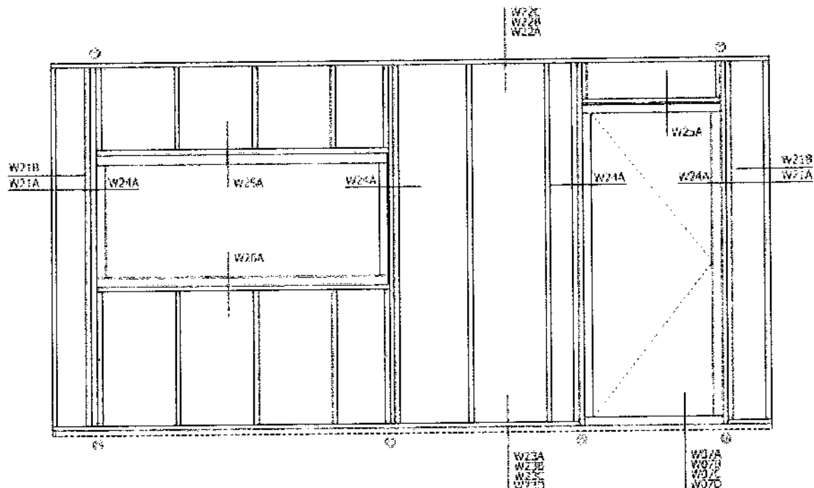
Details gevelvullende element- buitenzijde steenstrips
