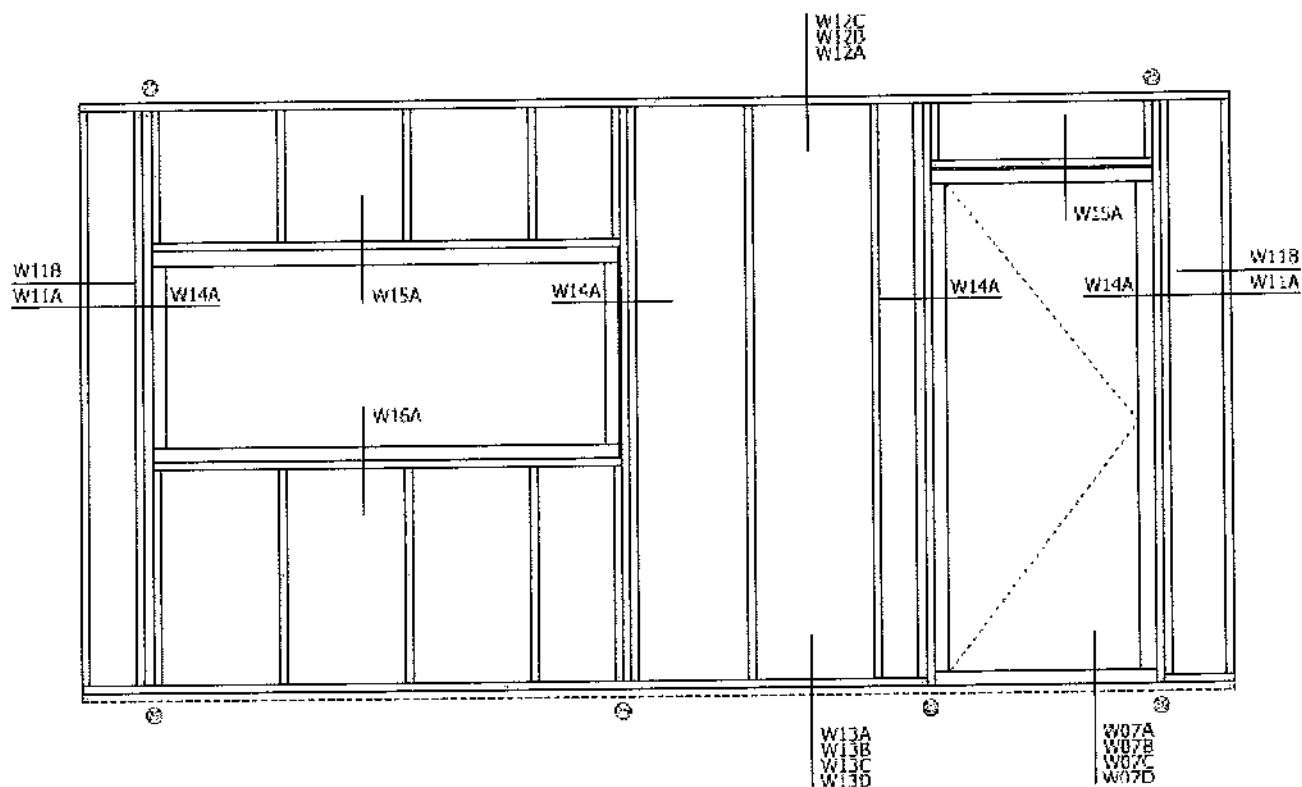
Details gevelvullende elementen – buitenzijde geveldelen
