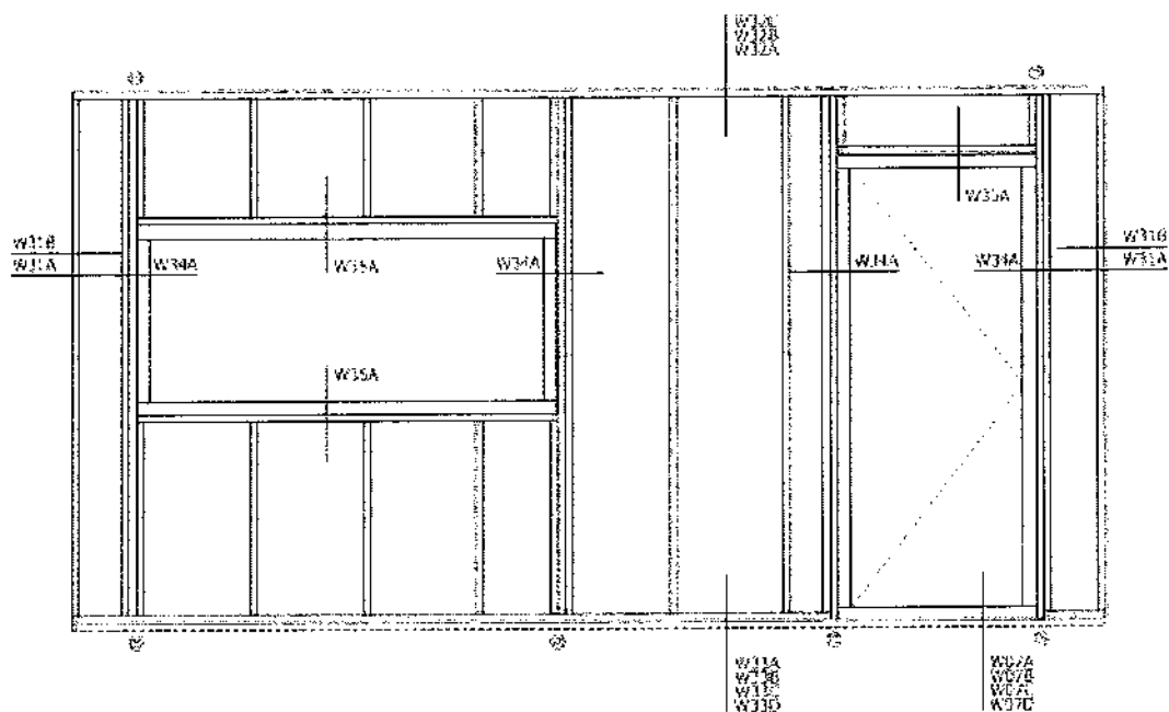
Details gevelvullende element – Buitenzijde gevelstuc
