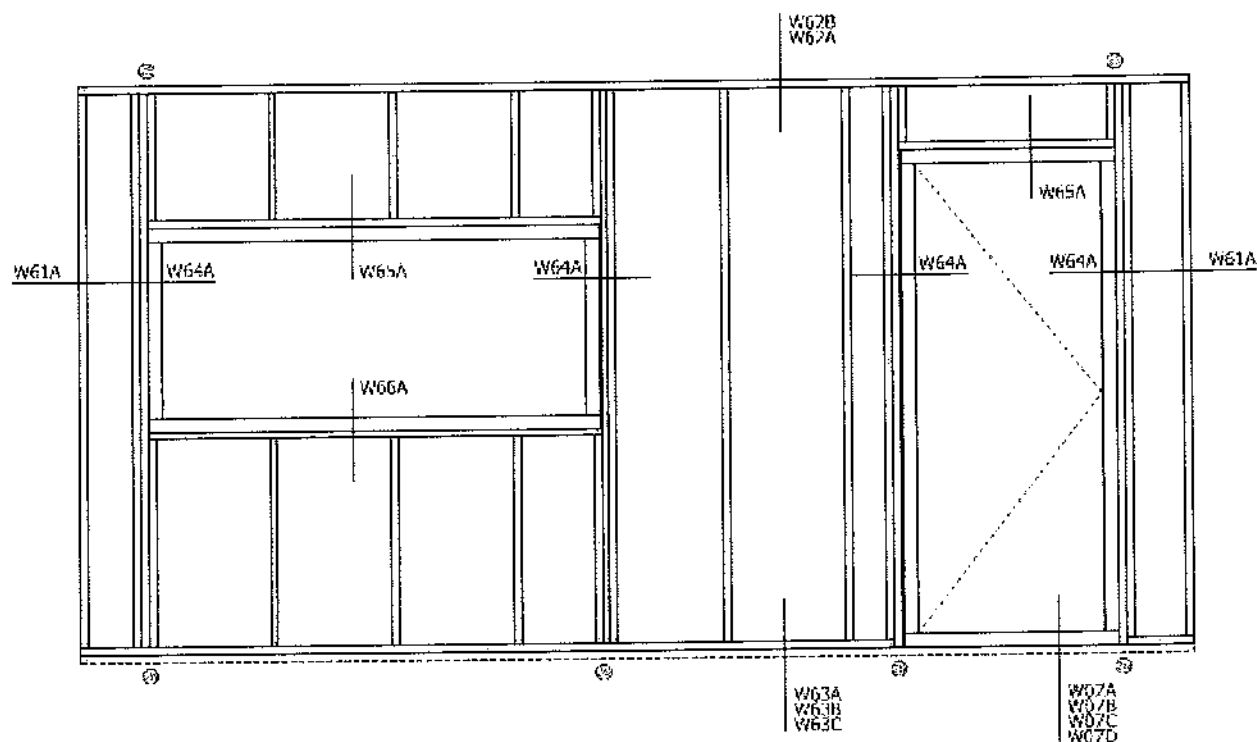
Details Voorzetwand - buitenzijde gevelstuc
