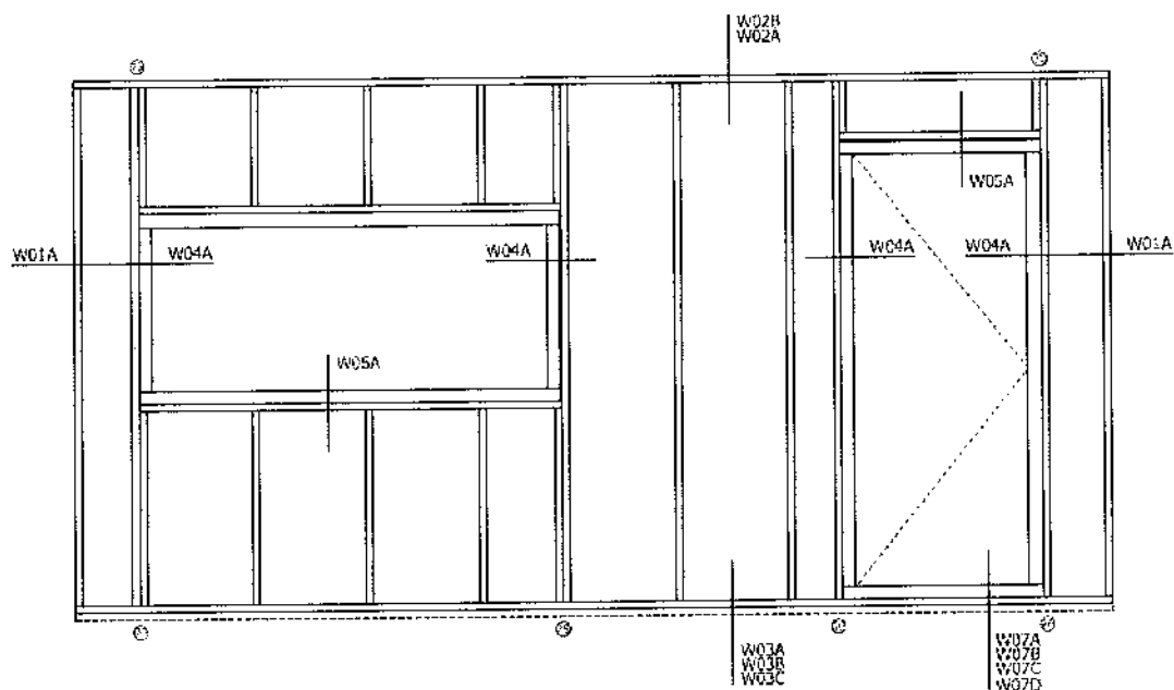
Details Binnenspouwblad (achter metselwerk)
