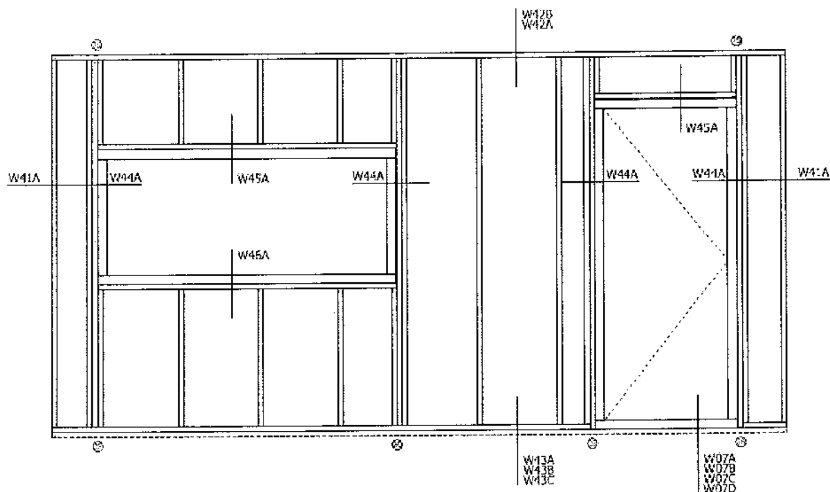
Details Voorzetwand - buitenzijde geveldelen
