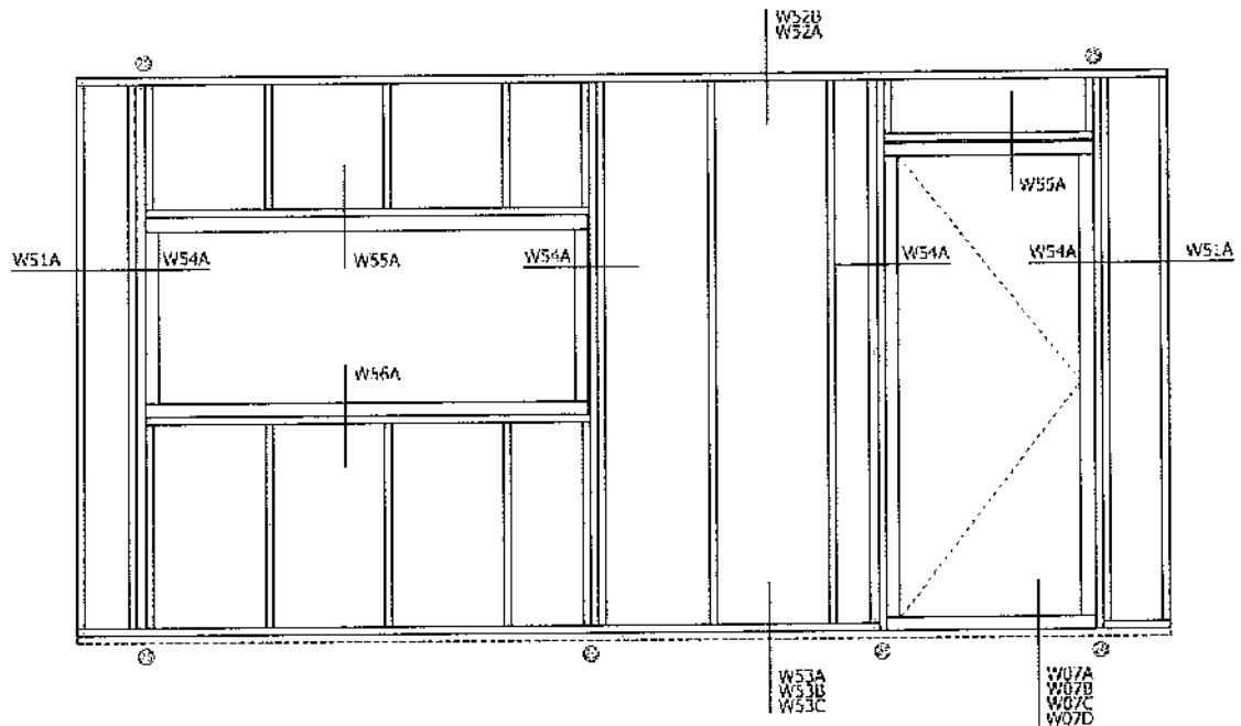
Details Voorzetwand - buitenzijde steenstrips
